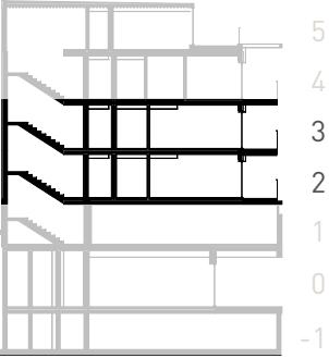
PISO 2 | 3
